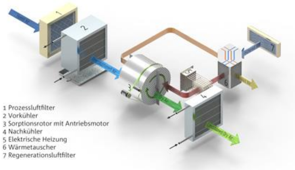
Bild 3: Beispiel eines Prozessluft-Trocknungsprozesses basierend auf Sorptionsverfahren
