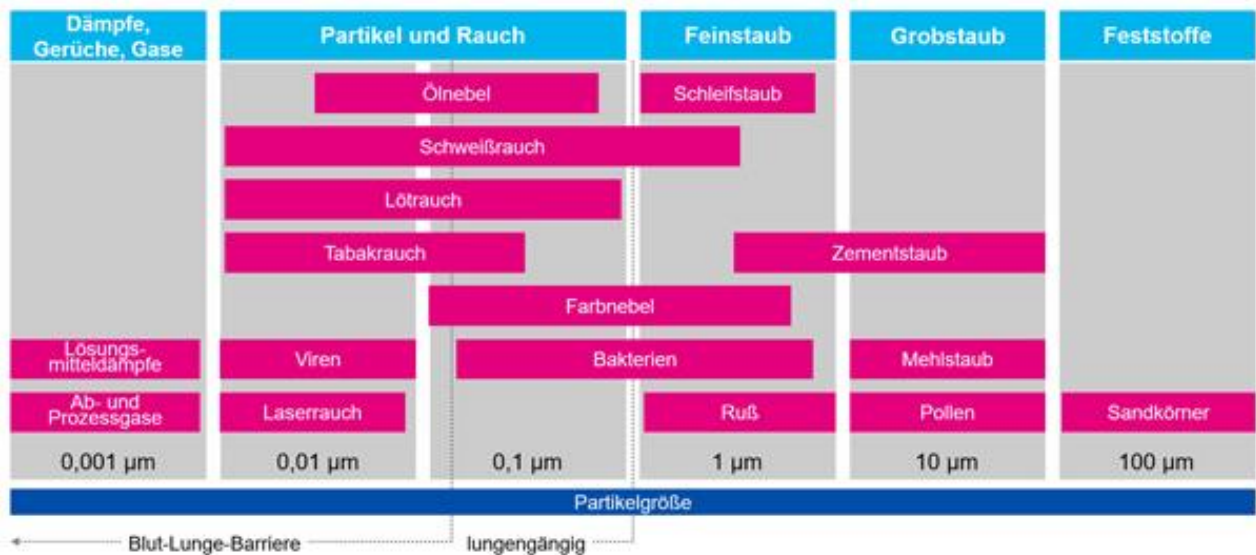
Bild 1: Übersicht über Staubpartikelgrößen
