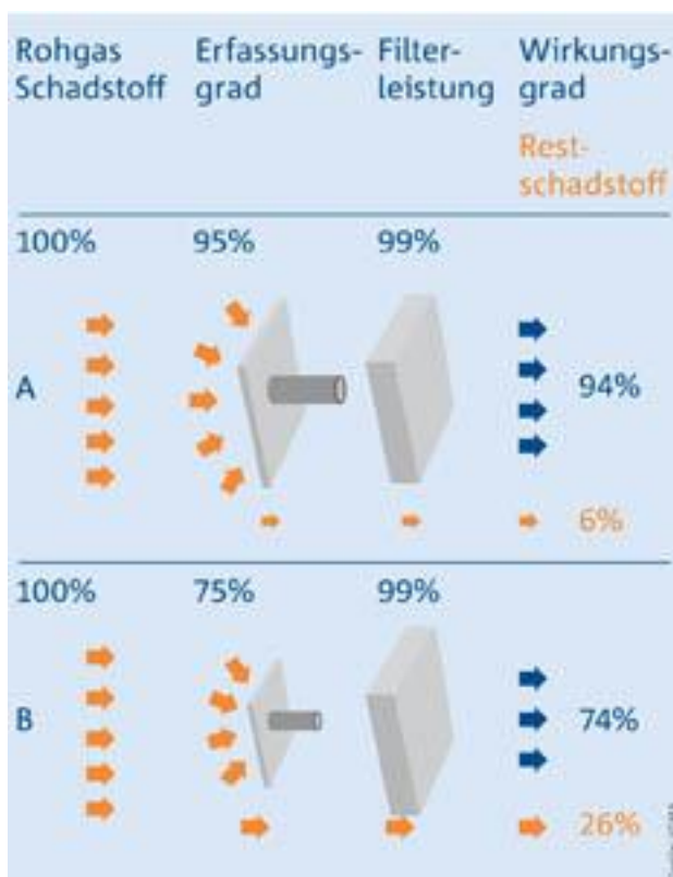
Bild 4: Reinigungsgrad im Verhältnis zum Erfassungsgrad
