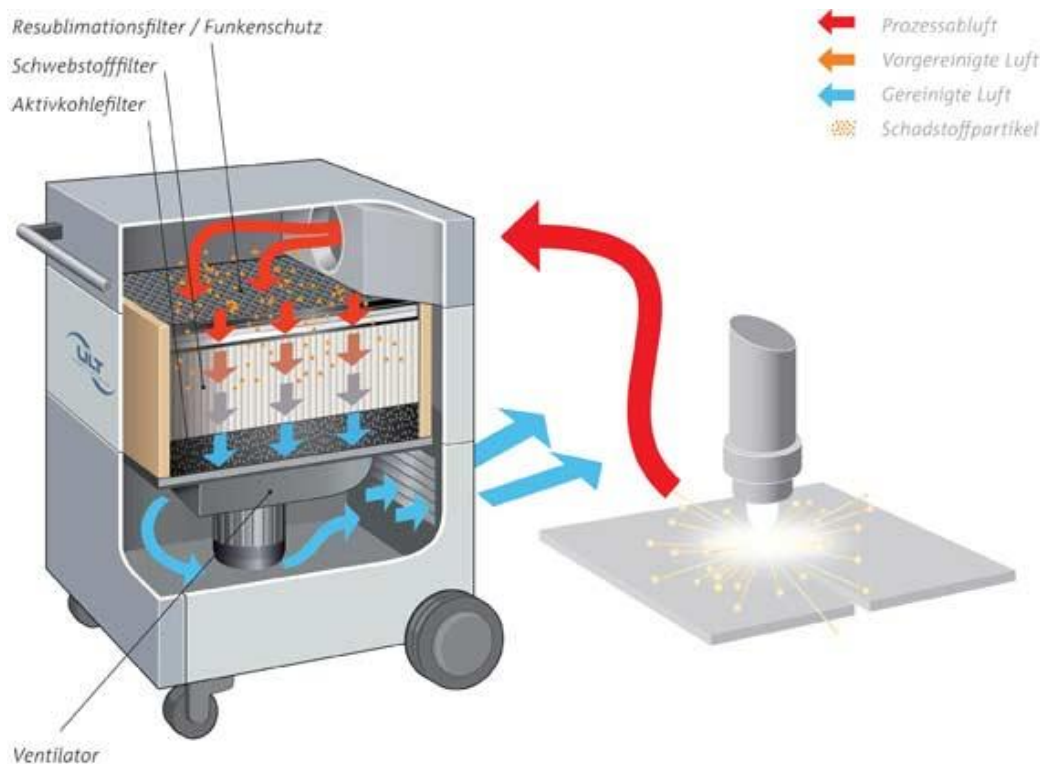
Bild 3: Beispiel Speicherfilter in einem Absaug- und Filtersystem für Laserprozesse
