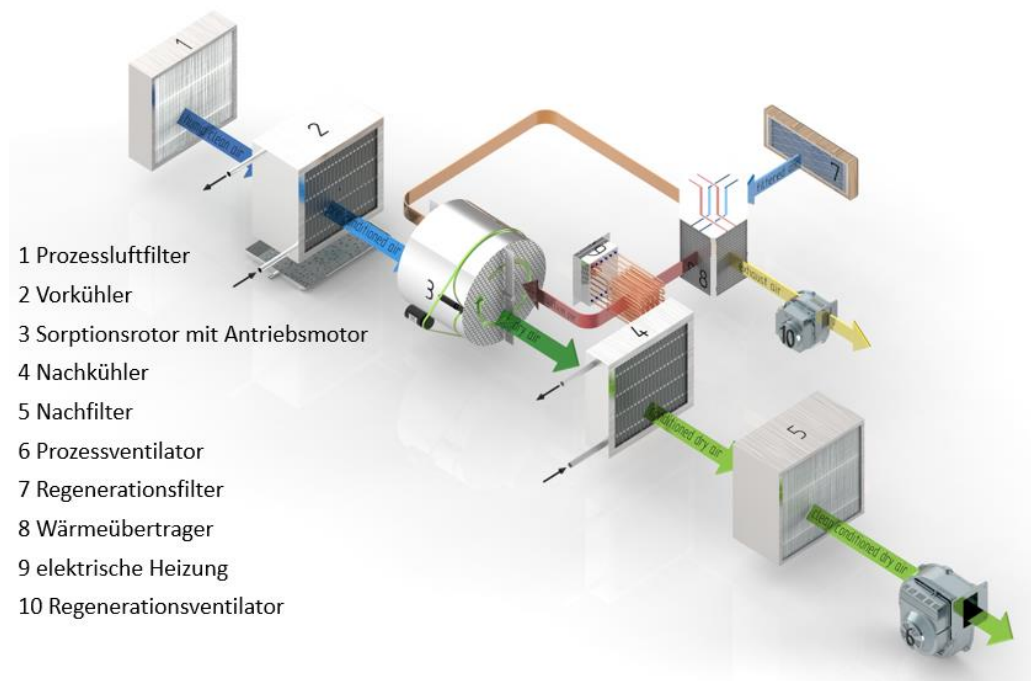
Bild 4: Bild 4: Lufttrocknungsprozess basierend auf Sorptionsverfahren
